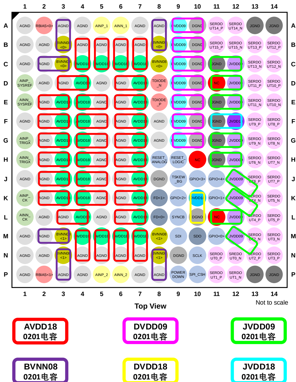
图 8-13. 推荐各电源滤波电容放置参考示意图
