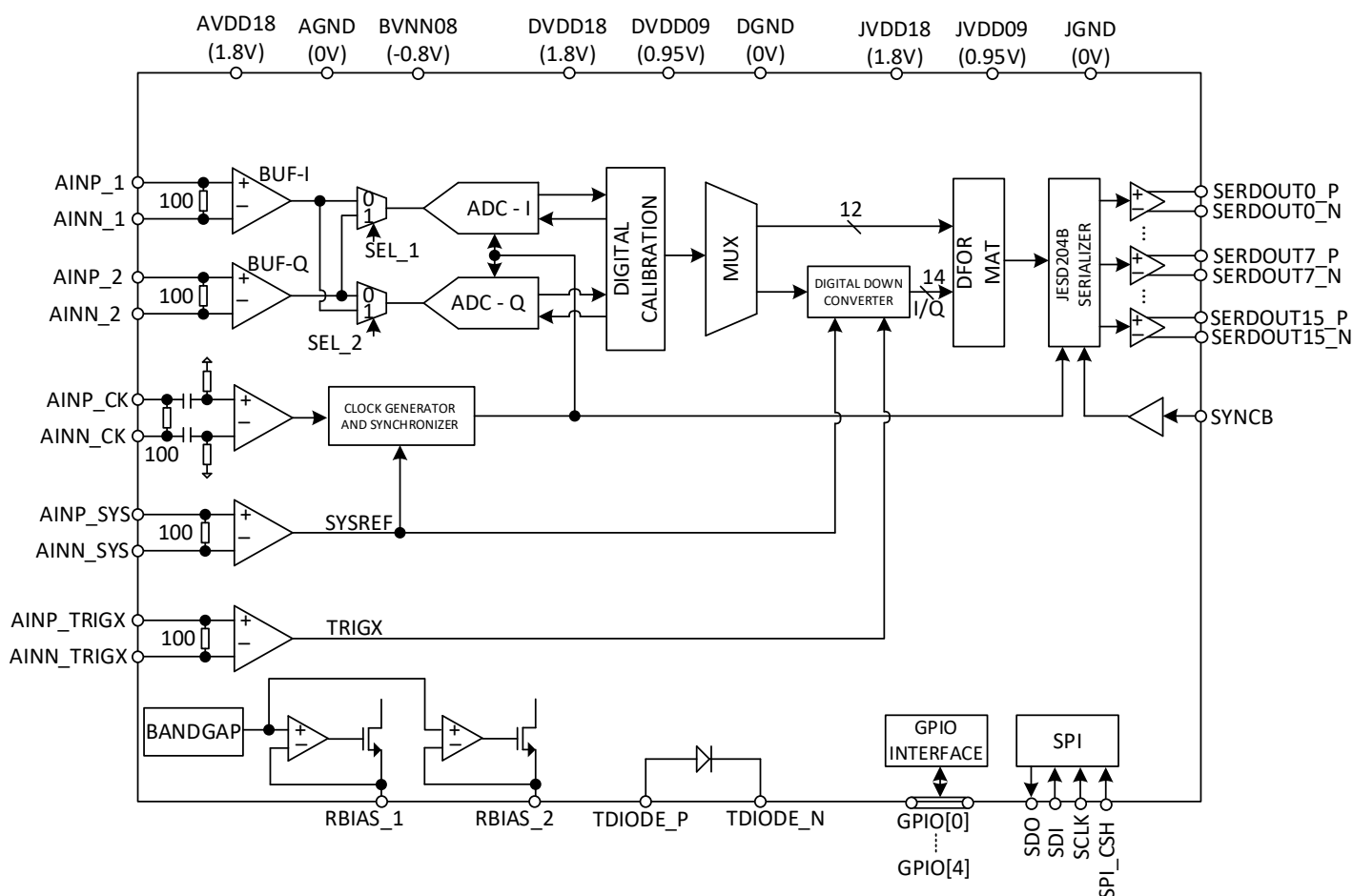
图 8-1. 功能框图
